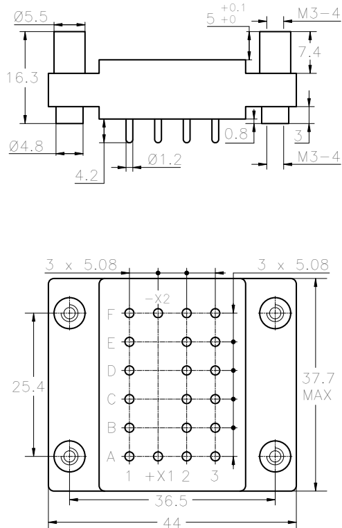
DIMENSIONS
